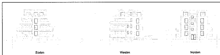
Abb. 7: Ansichten, geplantes Gebäude im S01 (Architekturbüro bielke und struve 07/2016)
