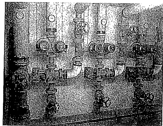
Ungeregelte Pumpengruppen
