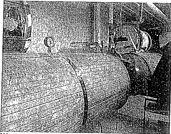
Wärmwasserspeicher 1000l
