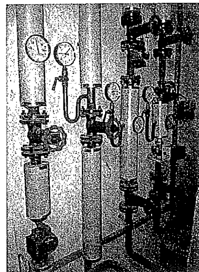
Heizverteiler Sporthalle
