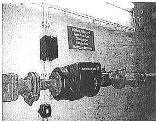
Heizkreispumpe geregelt
