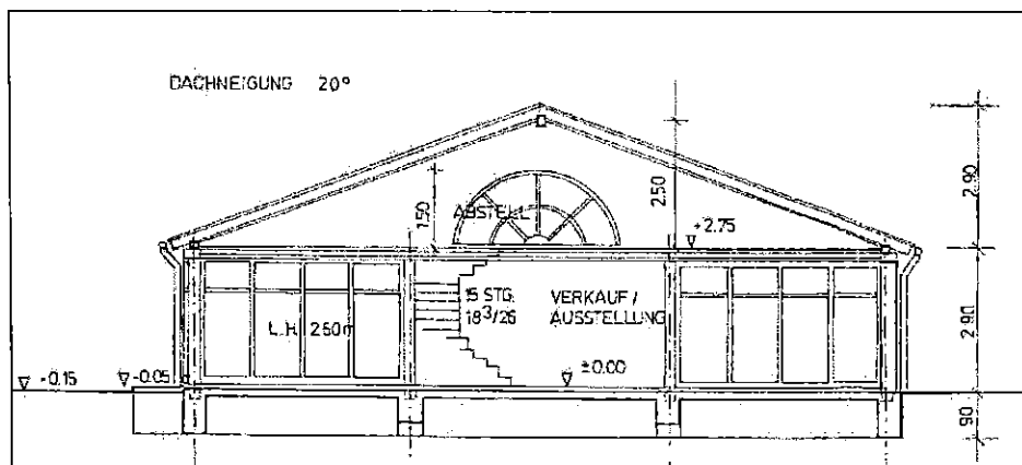
Abbildung 9: Prinzipschnitt Umnutzung Altbau
