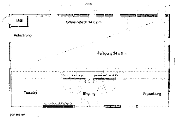
Abbildung 4: Prinzipdarstellung Grundriss EG Neubau Gläserne Erlebnissegelmacherei
