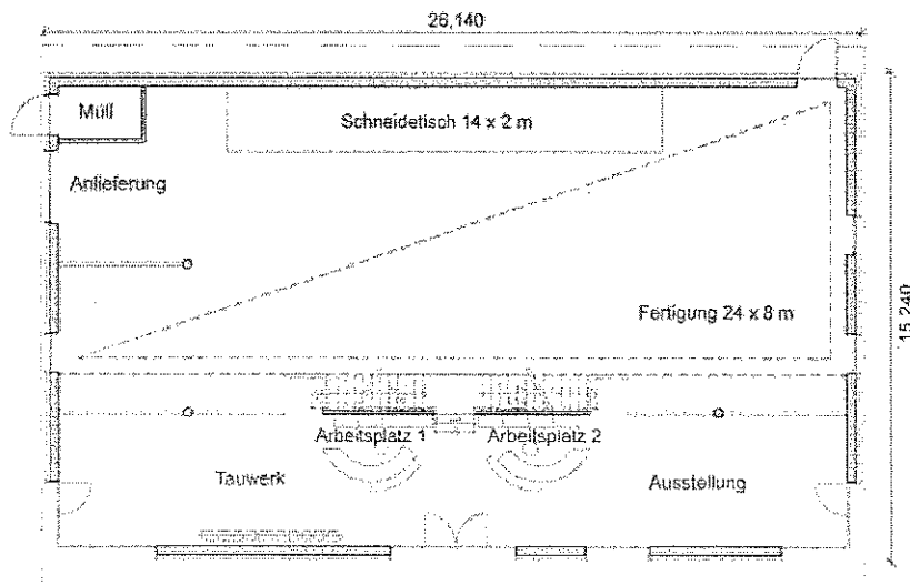
Abbildung 4: Prinzipdarstellung Grundriss EG Neubau Gläserne Erlebnissegelmacherei
