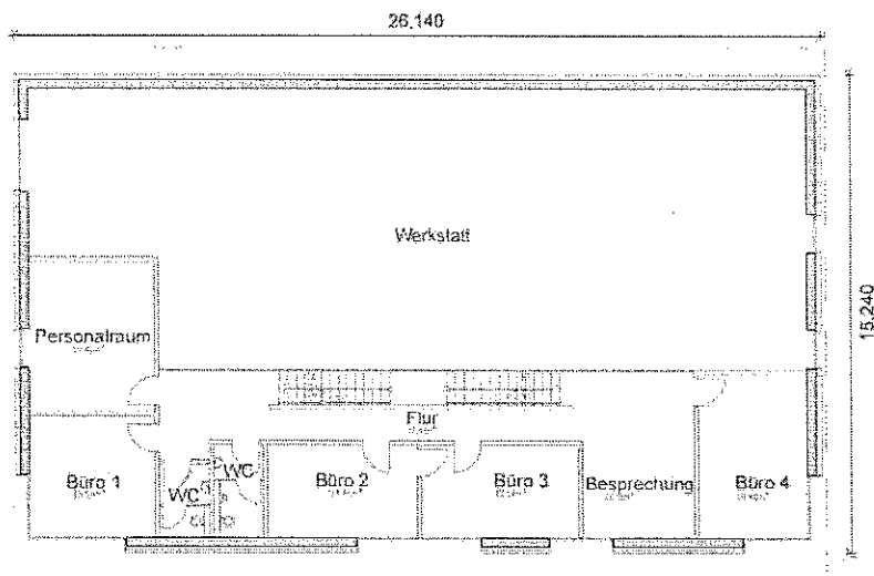
Abbildung 5: Prinzipdarstellung Grundriss 1.OG Neubau Gläserne Erlebnissegelmacherei
